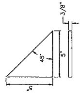
GUSSET PLATE SCALE: 3" = 1' - 0"
